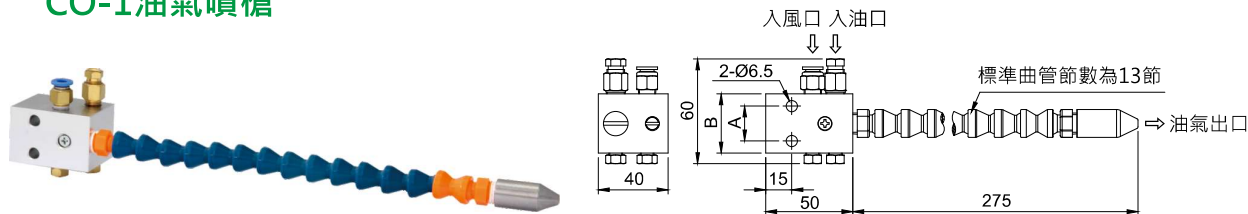
CO-1 油氣噴槍
