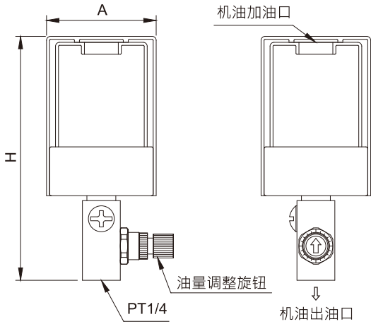
OP 外型图
