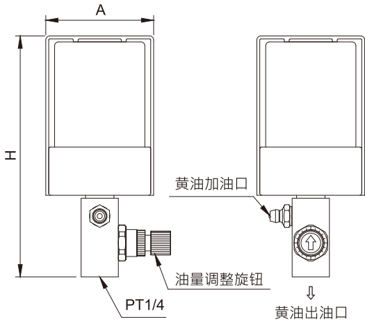
GP 外型图
